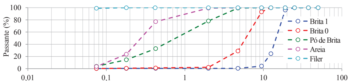
Figura 1: Distribuição granulométrica dos agregados convencionais
