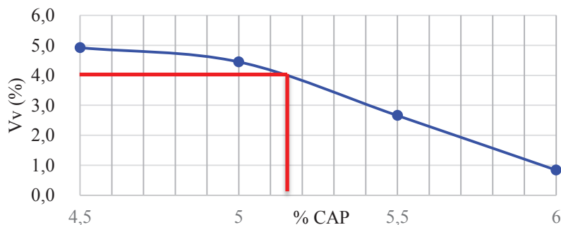
Figura 6: Análise gráfica do teor ótimo de ligante
