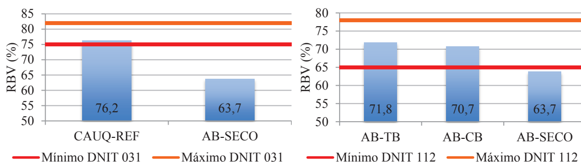
Figura 9: Valores da relação betume vazios (RBV)
