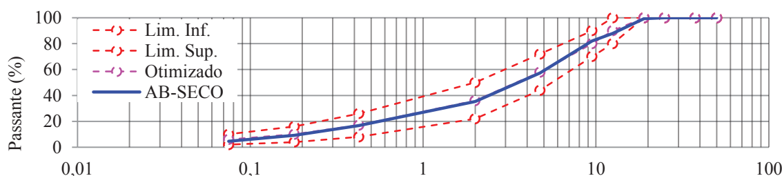
Figura 5: Enquadramento granulométrico da mistura asfálticas AB-SECO
