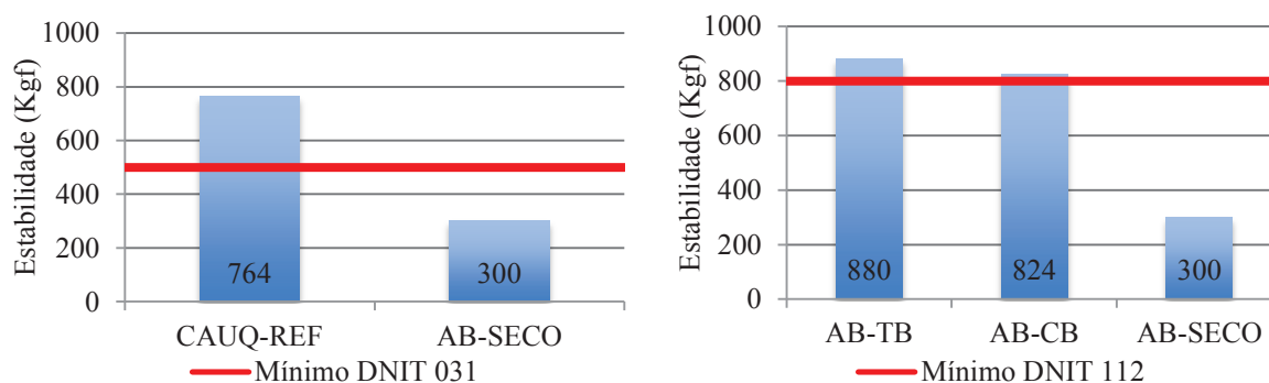
Figura 11: Valores da estabilidade Marshall
